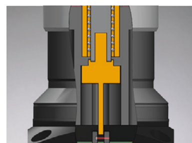
Le guidage linéaire à billes permet de faibles effort de mesure
