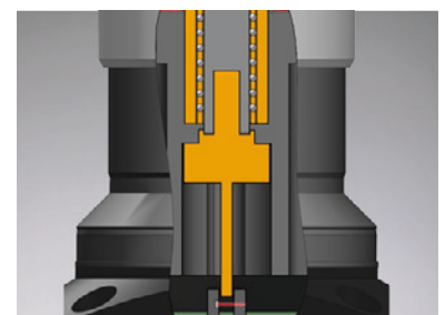
Die kugelgelagerte Linearführung ermöglicht geringe Messkräfte
