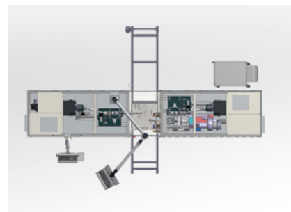
Layout mit Antrieb und Abtrieb rechts/links L = 5600 mm | B = 1100 mm
