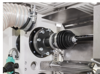
Fettaustrittsüberwachung und Fahrtwindsimulation
