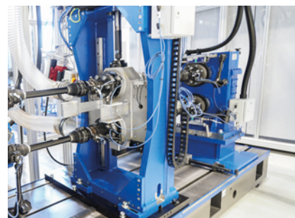
Pulsator für die Simulation einer Fahrstrecke
