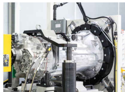
Prüfling adaptiert und gesichert während Prüfung
