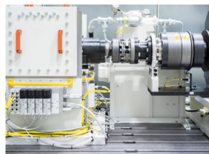
Sicherheitskupplung und Drehmoment-Messflansch im Antriebsstrang
