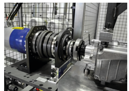
Antriebseinheit mit Drehmomentmessflansch
