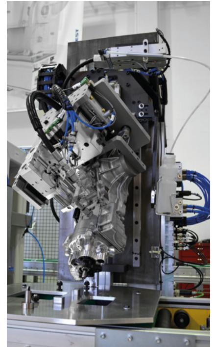
Ölbefüllung in optimaler Befülllage
