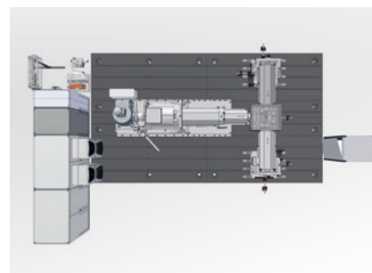
Mögliche T-Anordnung der Bremseinheiten
